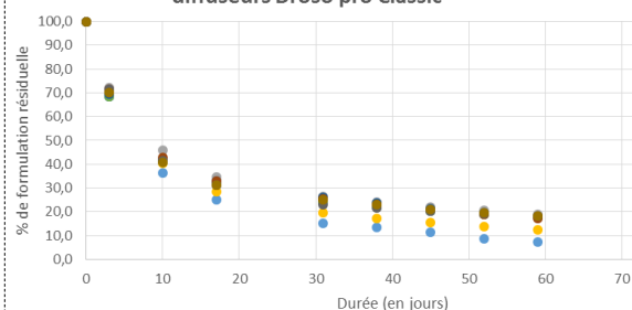
Cinétique de diffusion en étuve ventilée à 30°C de 4 diffuseurs Droso pro Classic
